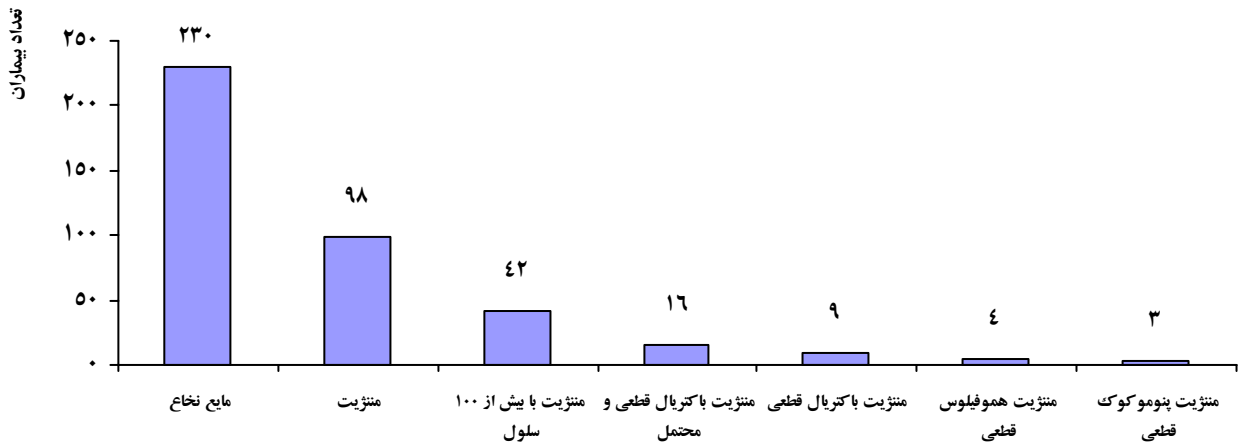
نمودار ۱- تجزیه کلی اطلاعات نمونه های مایع نخاع
