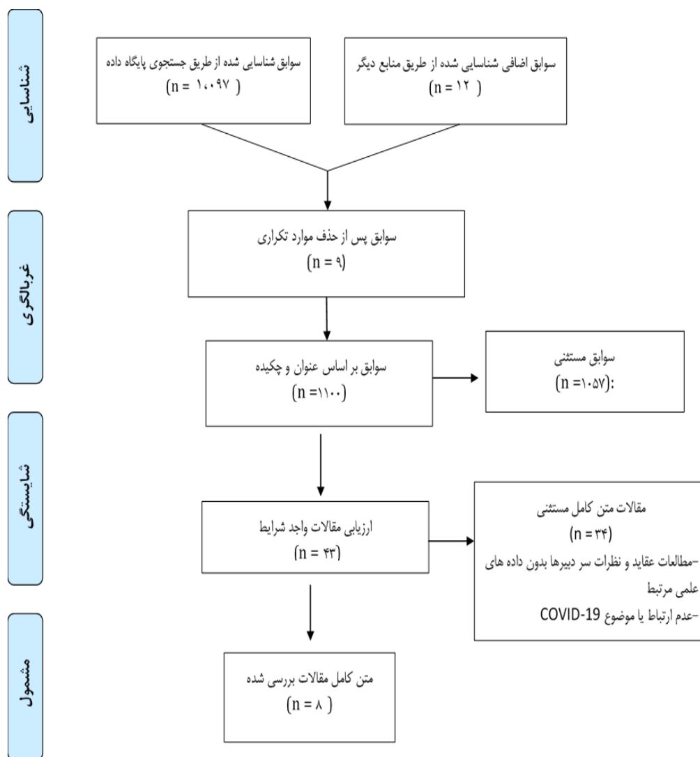
شکل ۱. نمودار PRISMA
