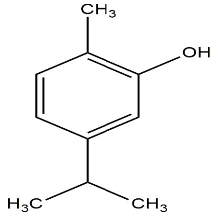
شکل ۱- ساختار شیمیایی کارواکروئل (۱۹).
